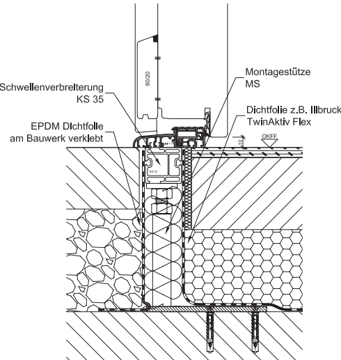
Detail Fußpunkt
