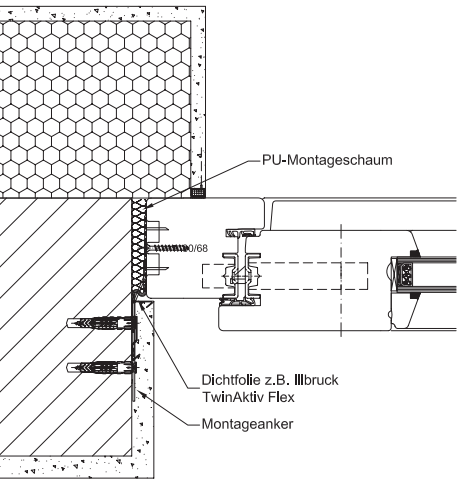
Detail seitlich
