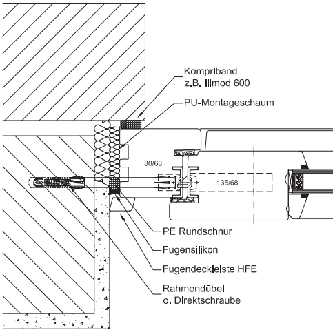
Detail seitlich
