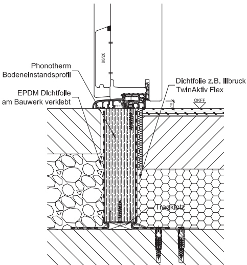
Detail Fußpunkt
