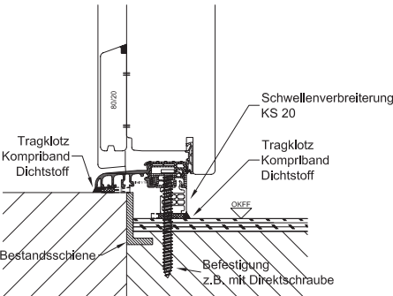
Detail Fußpunkt
